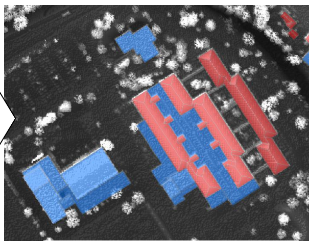
Für die Potentialberechnungen erkannte Dachseiten (rot = Spitzdach / blau = Flachdach)
